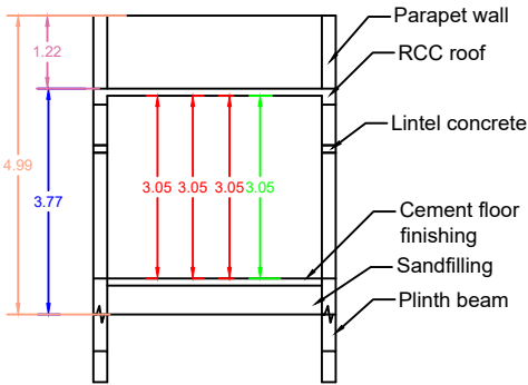
SECTION - AB
