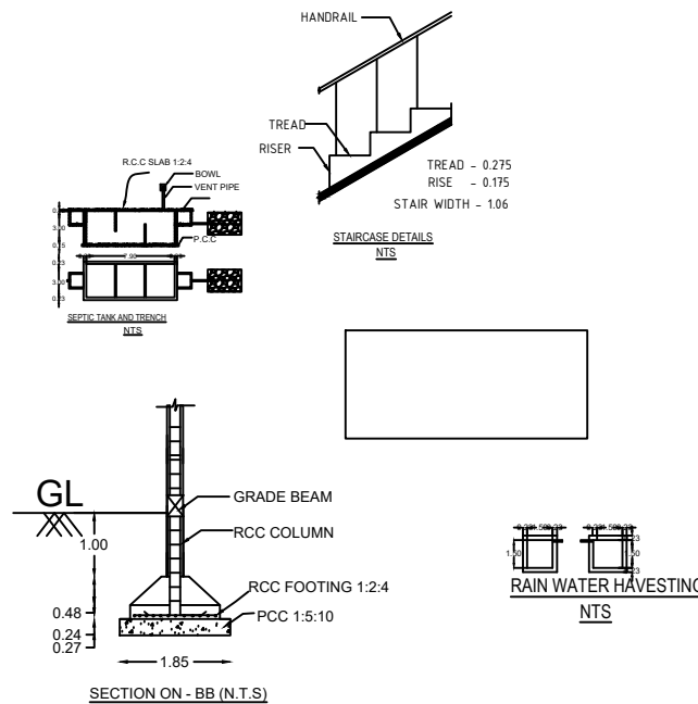
SECTION ON - BB (N.T.S)
