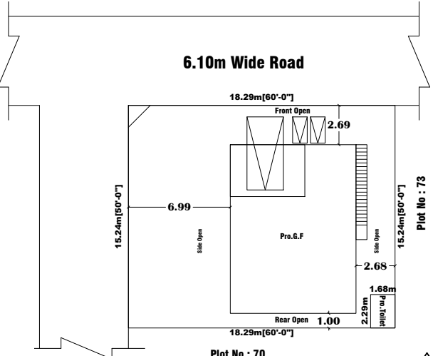
Plot No : 70 Site Plan (Scale 1:200)
