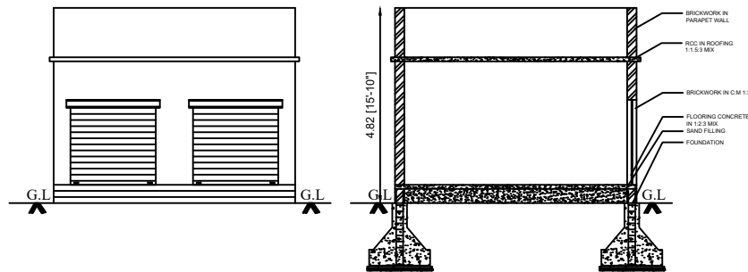
ELEVATION
