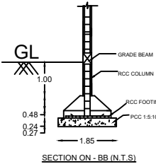
SECTION ON - BB (N.T.S)
