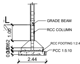
SECTION ON - BB (N.T.S.)
