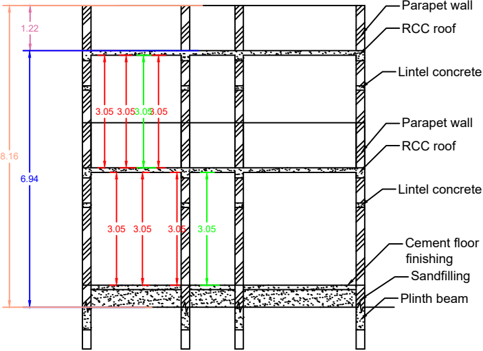
SECTION - AB
