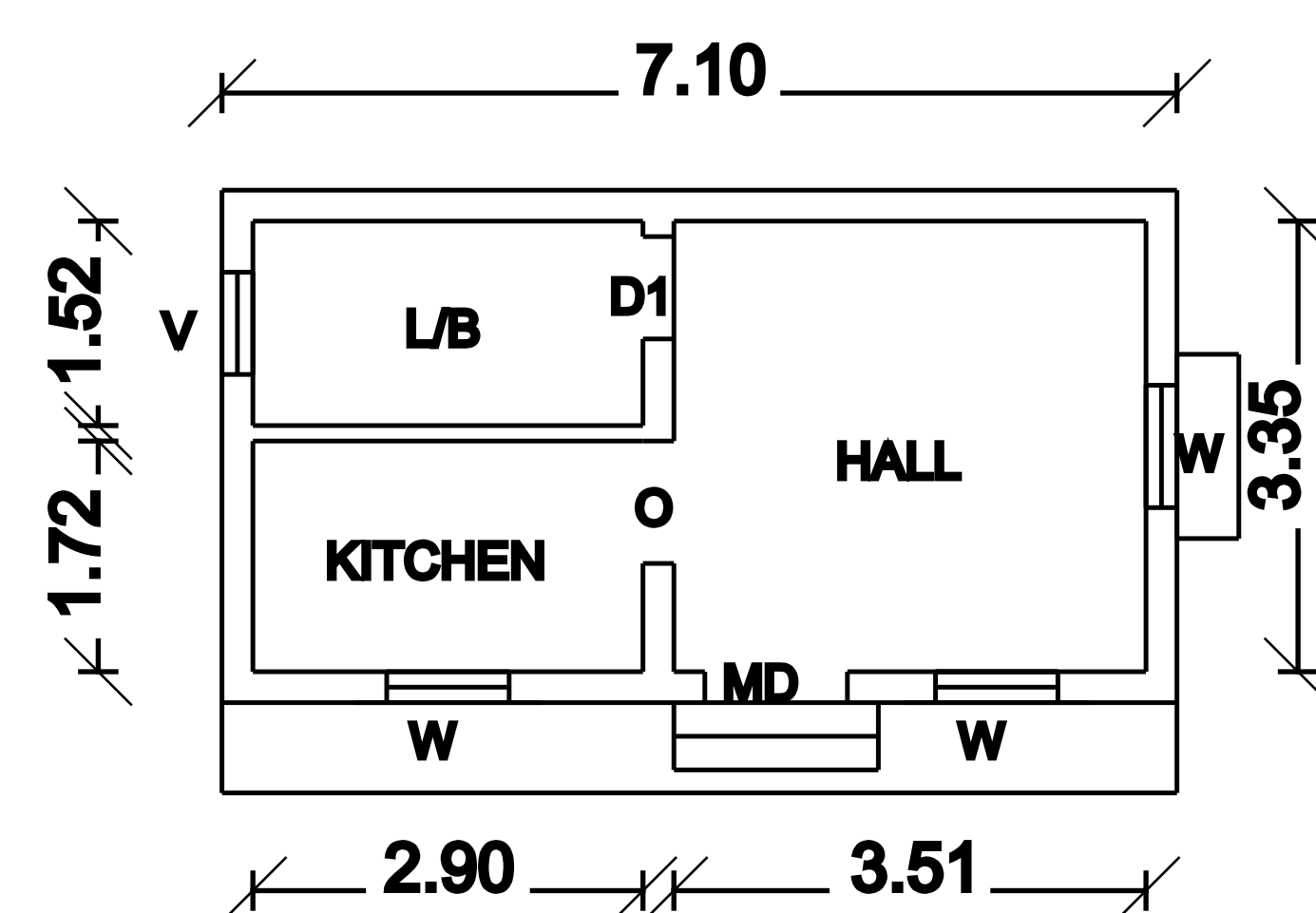
G.F PLAN
