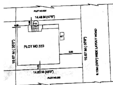
SITE PLAN SCALE: 1:200
