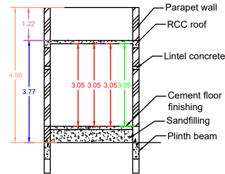
SECTION - AB
