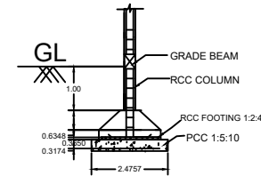
SECTION ON - BB (N.T.S)
