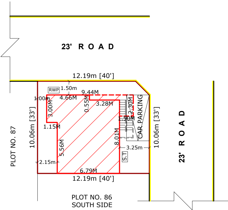
SITEPLAN (SCALE: 1:200)
