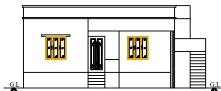
ELEVATION
