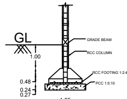
SECTION ON - BB (N.T.S)
