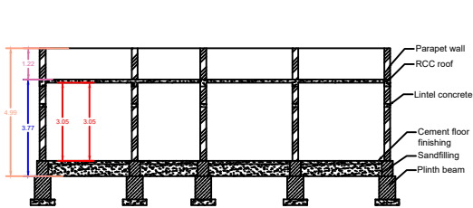
SECTION - AB
