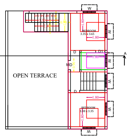
F.F PLAN
