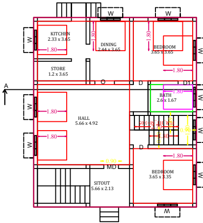
G.F PLAN
