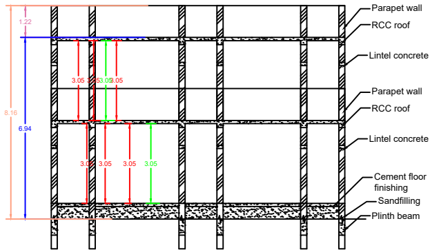
SECTION - AB
