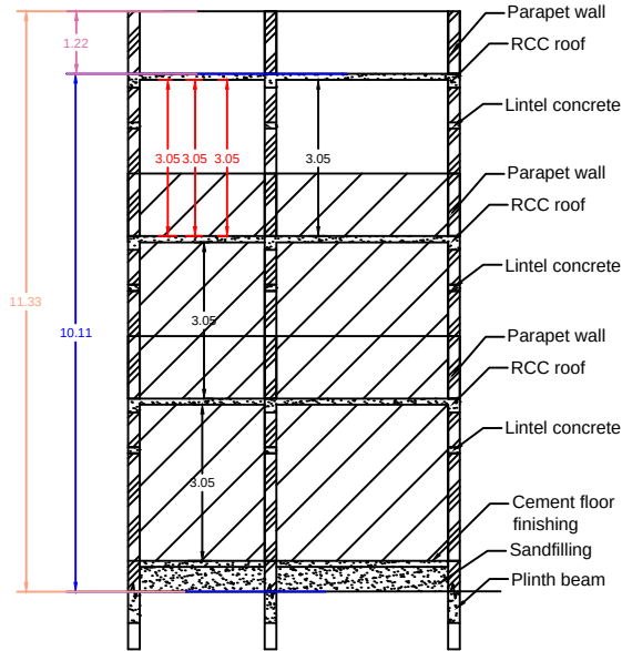
SECTION - AB
