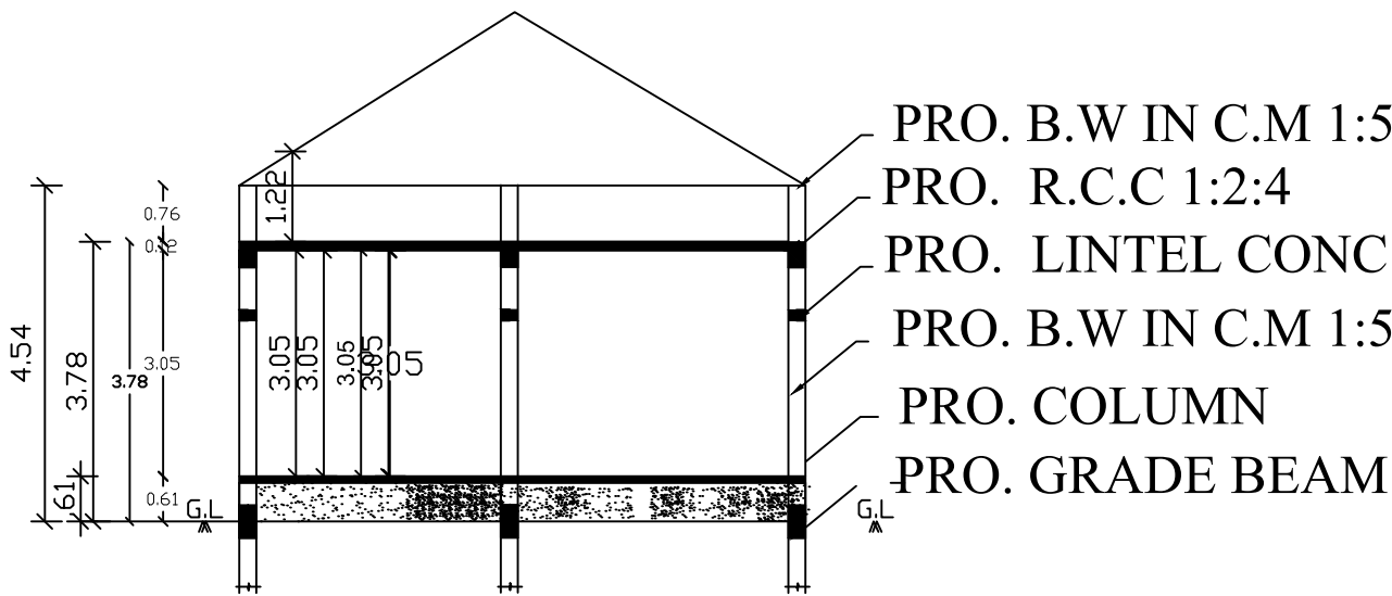
ELEVATION
