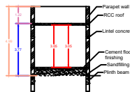
SECTION - AB
