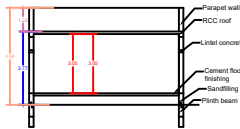
SECTION - AB
