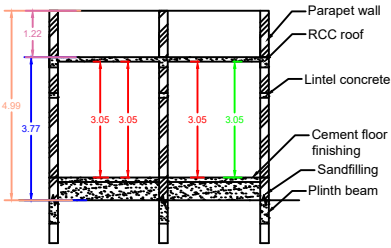
SECTION - AB
