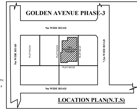
SITE PLAN(SCALE 1:100)
