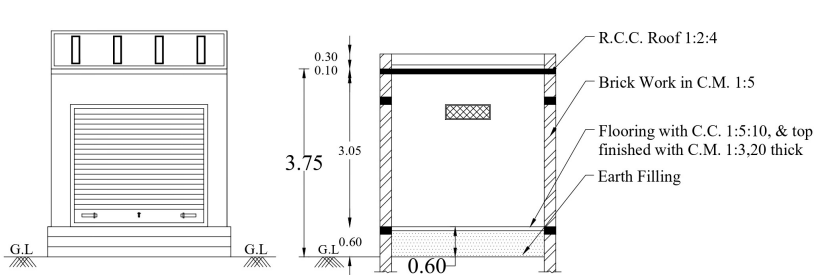
ELEVATION
