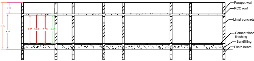
SECTION - AB
