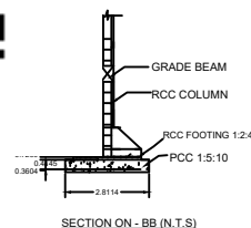
SECTION ON - BB (N.T.S)
