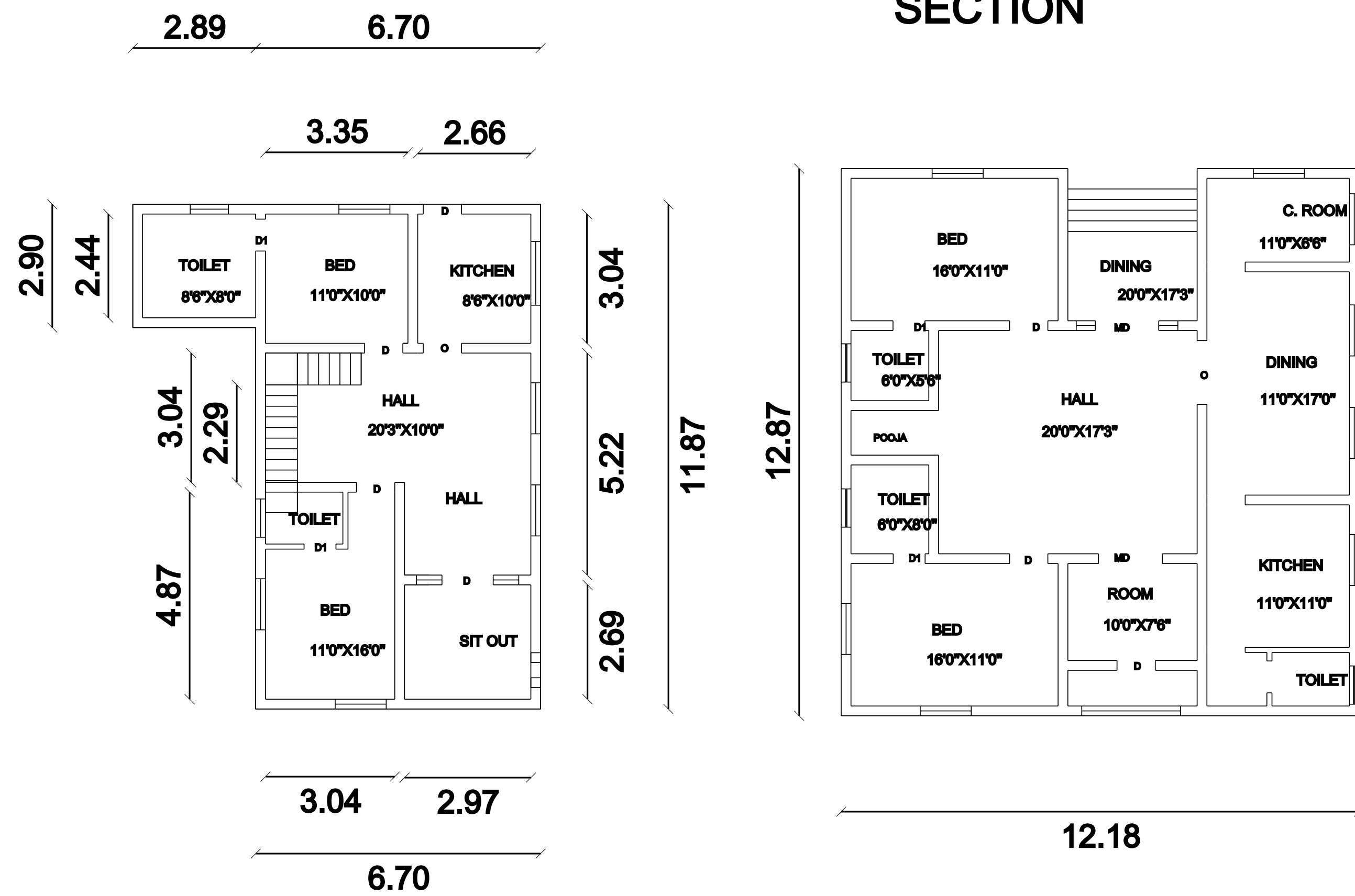
EXISTING D.NO 15/327 HOUSE PLAN
