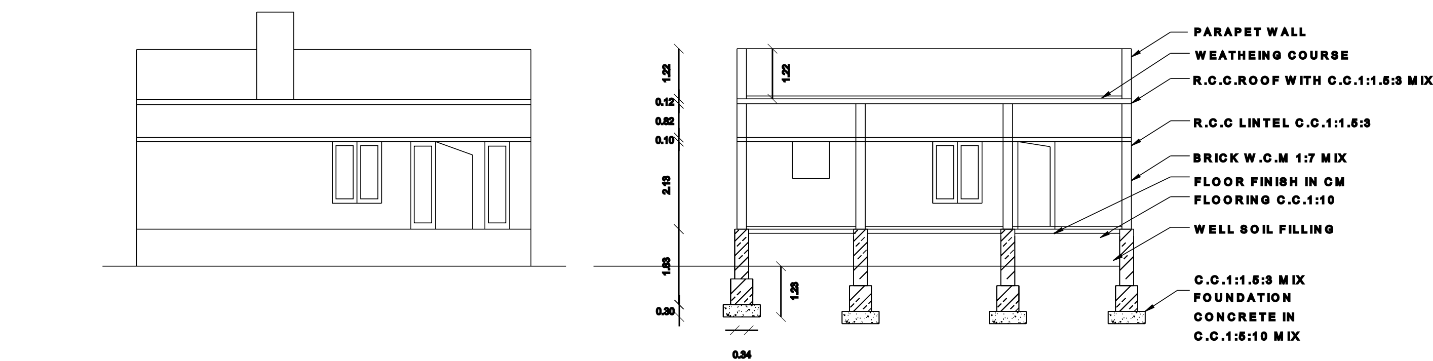
ELEVATION
