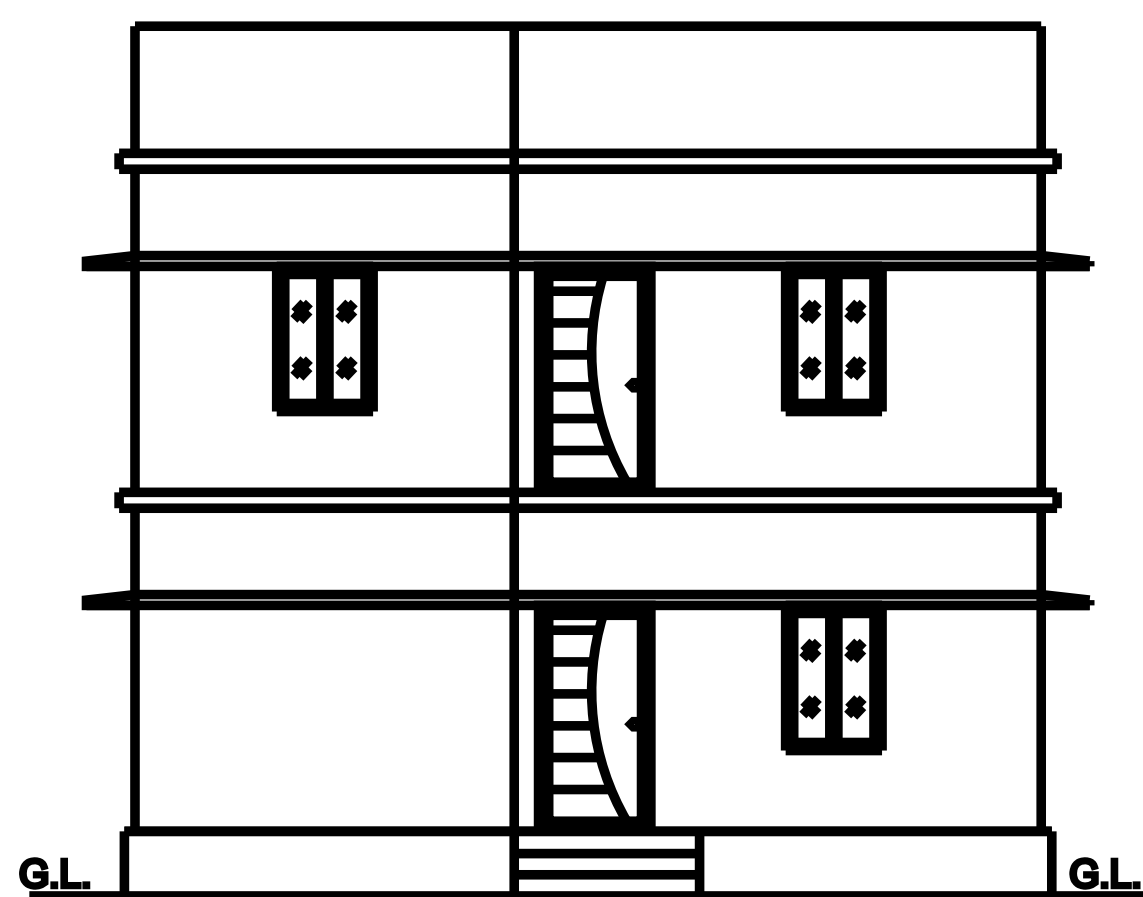
ELEVATION
