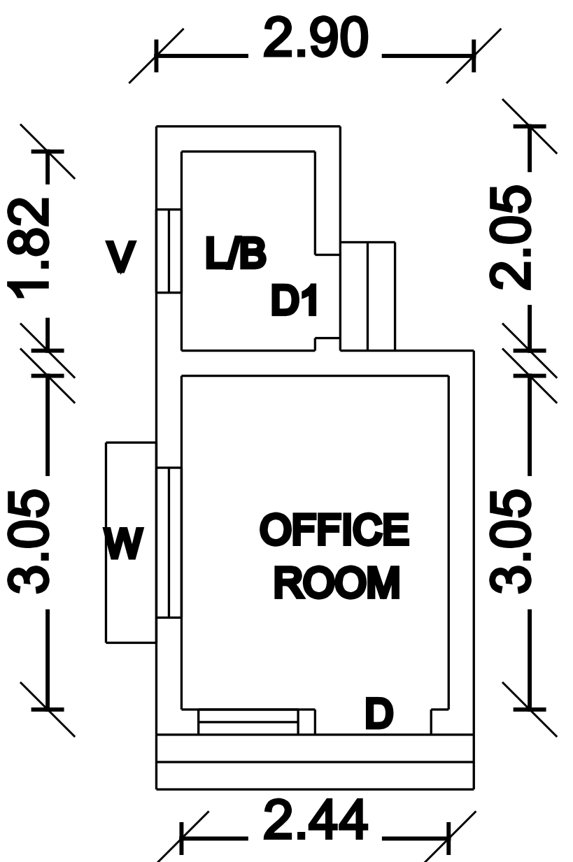
G.F PLAN
