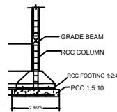
SECTION ON - BB (N.T.S.)
