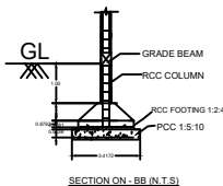
SECTION ON - BB (N.T.S)
