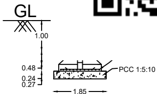
SECTION ON - BB (N.T.S)
