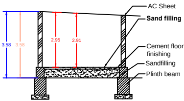
SECTION - AB
