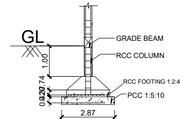
SECTION ON - BB (N.T.S)
