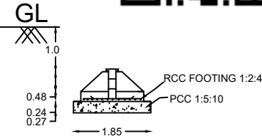
SECTION ON - BB (N.T.S)
