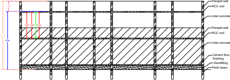
SECTION - AB
