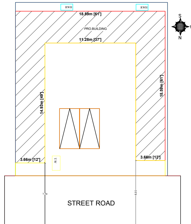
SITE PLAN 1:100 SCALE
