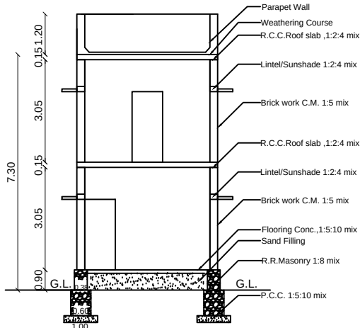
SECTION A-B
