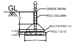
SECTION ON - BB (N.T.S)
