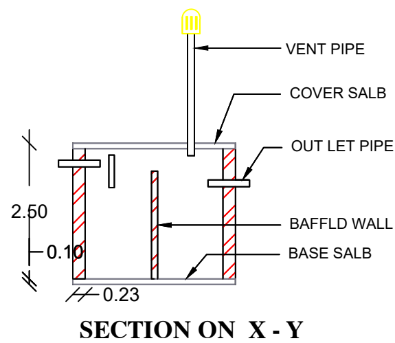
SECTION ON X - Y
