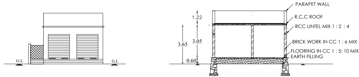
ELEVATION
