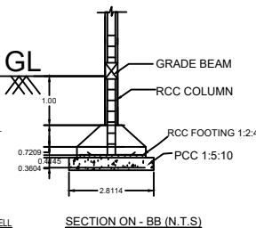
SECTION ON - BB (N.T.S.)
