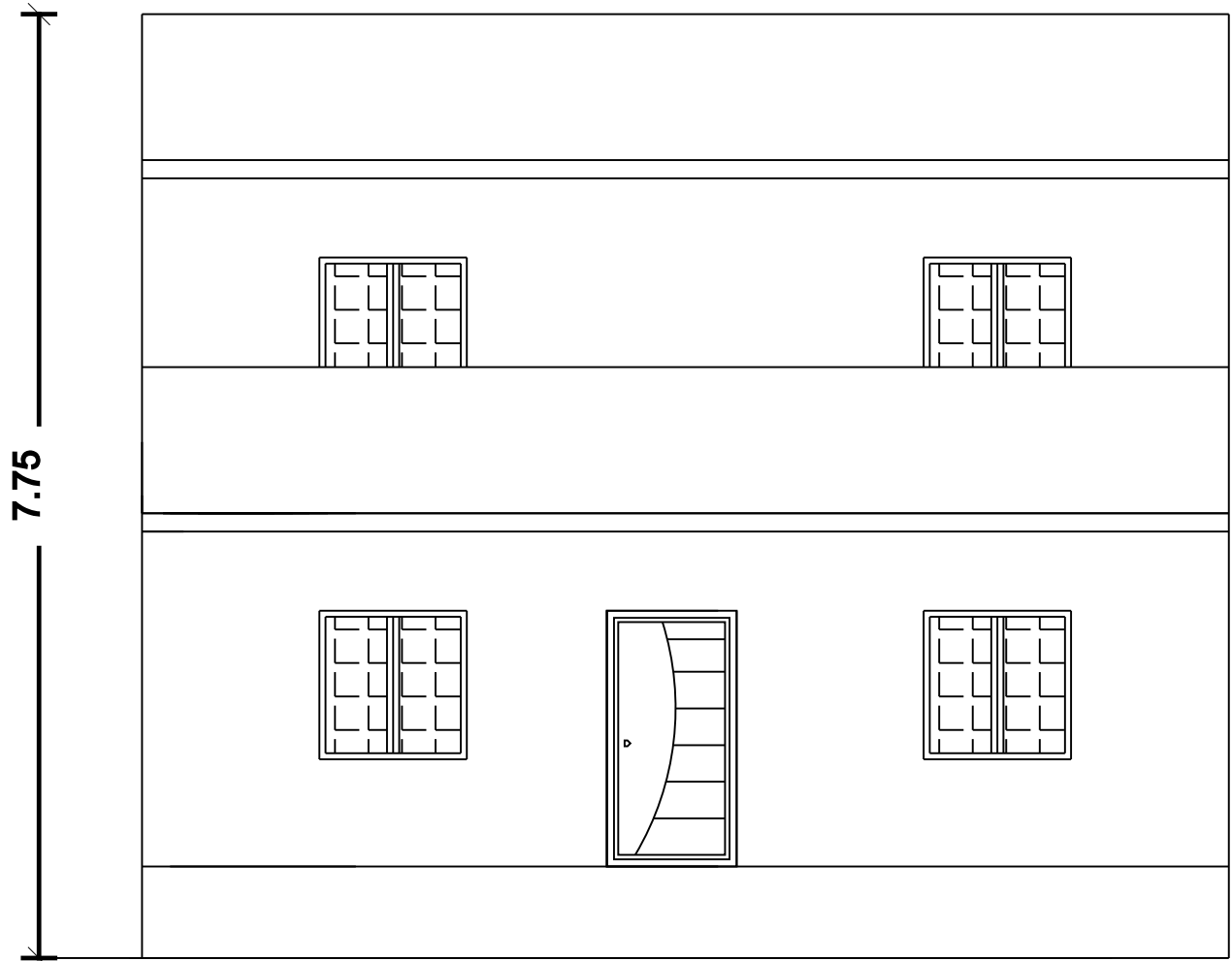
ELEVATION
