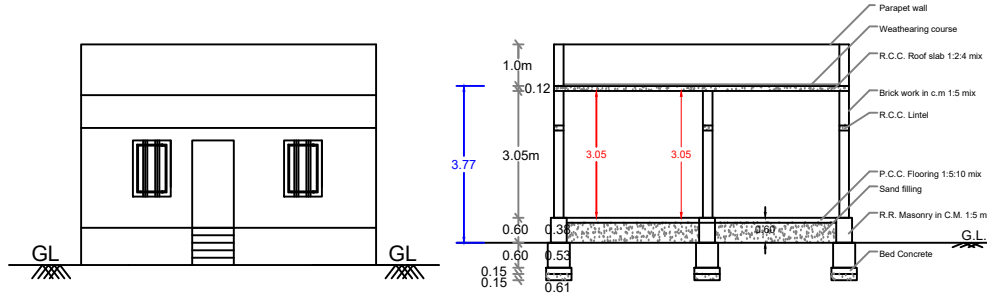
ELEVATION
