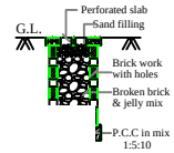
SEPTIC TANK (SCALE)
