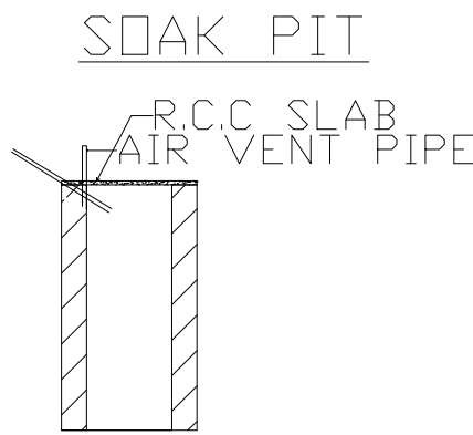
SOAK PIT
