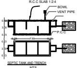
SEPTIC TANK AND TRENCH N.T.S
