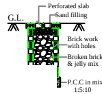
ION PIT (SCALE)
