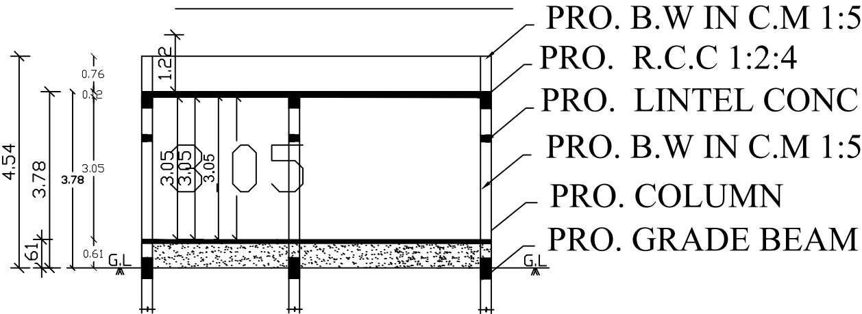
ELEVATION
