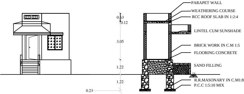
ELEVATION - 1
